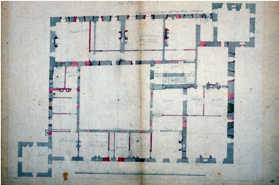
Plattegrond van de tweede verdieping van Neubourg door Johann Joseph Couven. De kleuren zijn versterkt. Suermondt-Ludwig-Museum Aachen, CBK 48. Foto Wolfgang von Gliszczyński.
