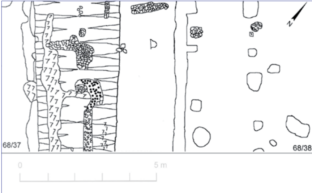
Afb. 24 Opgravings-tekening Xanten met gracht (links) en funderingsleuf met rechts daarvan (onder andere) een palenrij. Bron: Müller et al., 2008, afbeelding 85.
