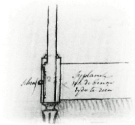
II p. 110B bevestiging van hoofd- en voeteneinde aan het zijschot met behulp van een schroef.
