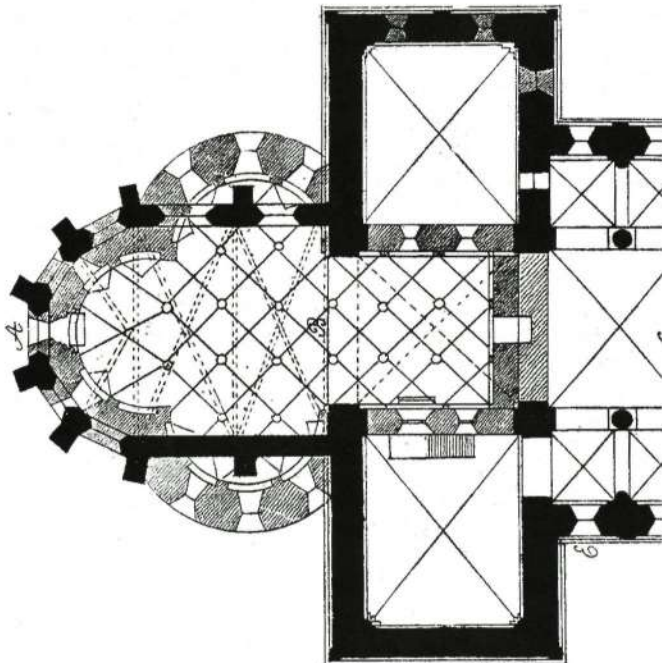
Plattegrond van koor en crypte volgens F. Bock in 1859; rechts in de brede westelijke muur van de crypte de "confessio".
