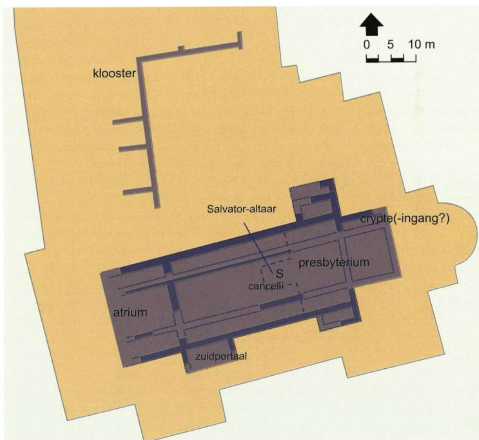
Afb. 10. Maastricht, St.-Servaaskerk. Contouren van de huidige kerk met de ligging van de laat-Merovingische basilica (blauw) en enkele muurresten van een vroege kloosterbouw in de pandtuin (lichter blauw) (tekening: auteur).
